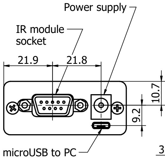
IR module socket D-sub 9 pin (female)
